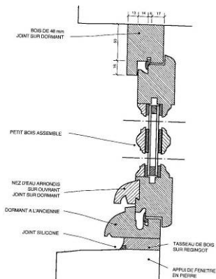
Coupe
